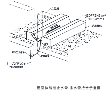
屋面伸縮縫止水帶-排水管接合示意圖
